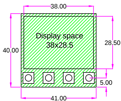
COMPONENTS P.C.B - 3 40X41
