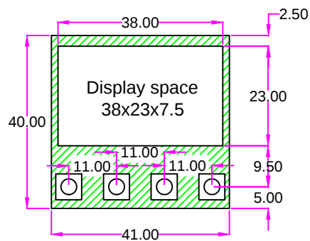
COMPONENTS P.C.B - 3 40X41
