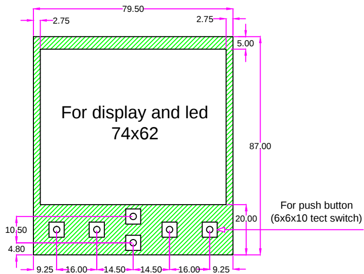
P.C.B no:1 size 79.5x87 Display P.C.B card
