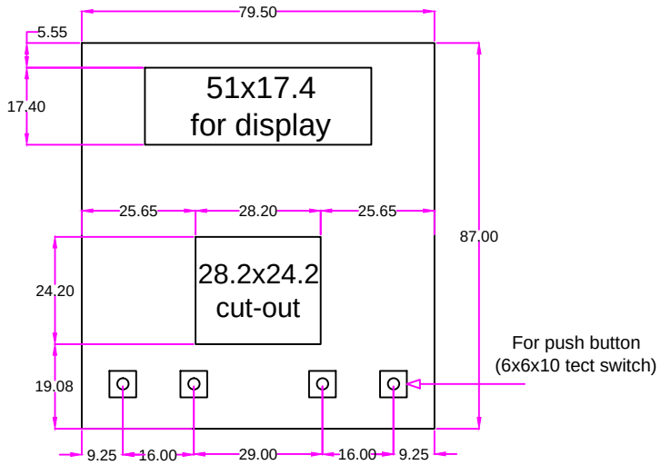
P.C.B no:1 size 79.5x87 Display P.C.B card
